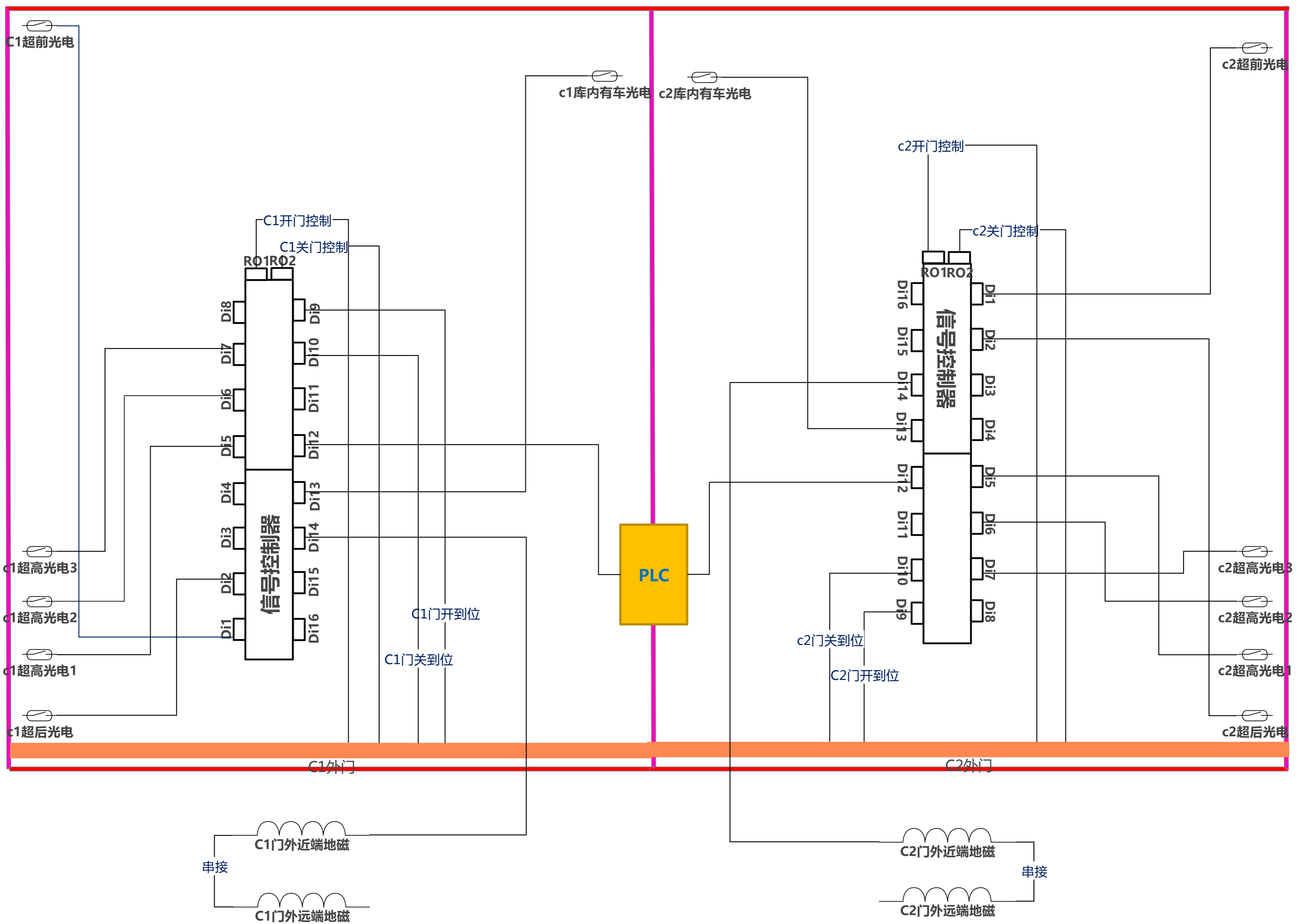
入口传感器系统图
