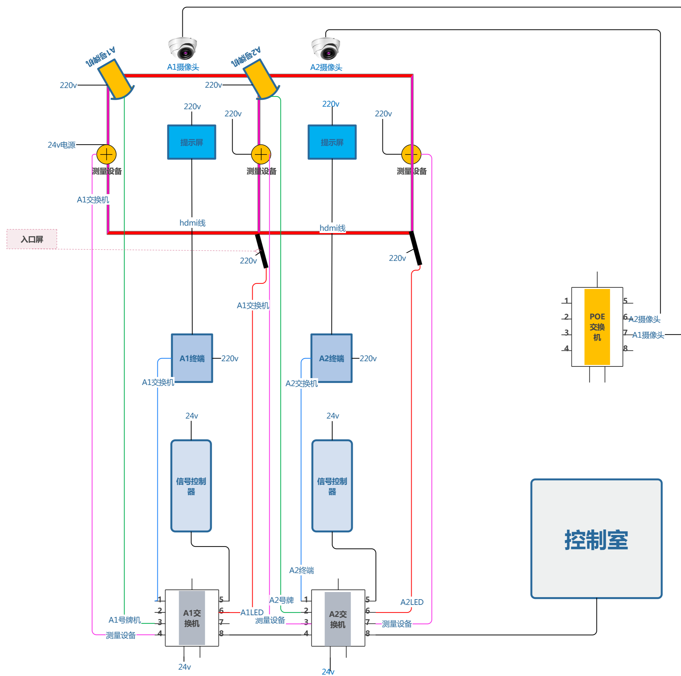
入口交互及测量设备系统图
